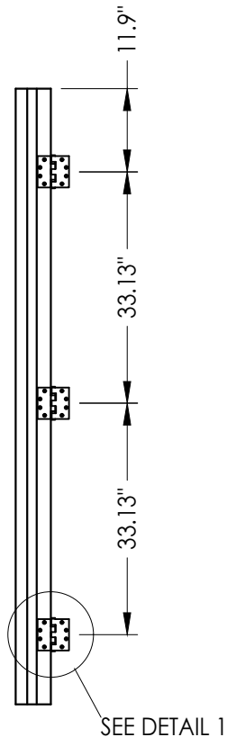
HINGE JAMB
